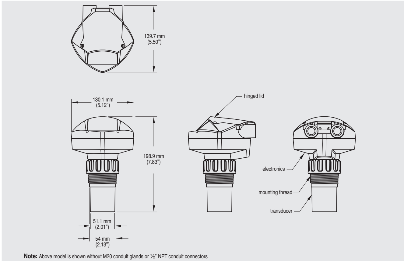
Fig. 4/2 SITRANS Probe LU dimensions
